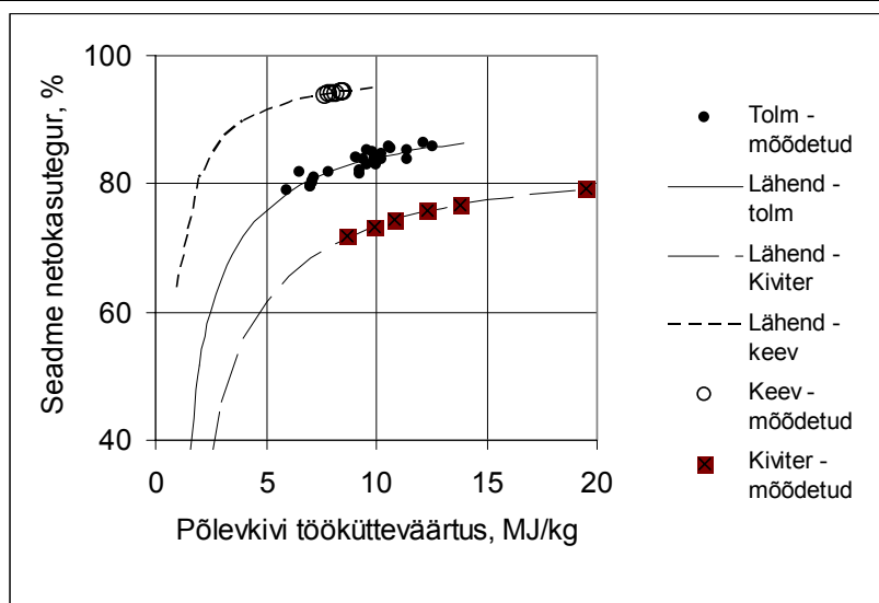
Pilt 3.4. Kõige üldisem seos põlevkivi kasutatavate seadmete kasuteguri ja põlevkivi kütteväärtuse vahel. Tolm – põletamine tolmküttekateldes, Keev – põletamine keevkihtkateldes, Kiviter – õli utmine gaasigeneraatorites, Lähend – kirjeldava funktsiooni graafik.
